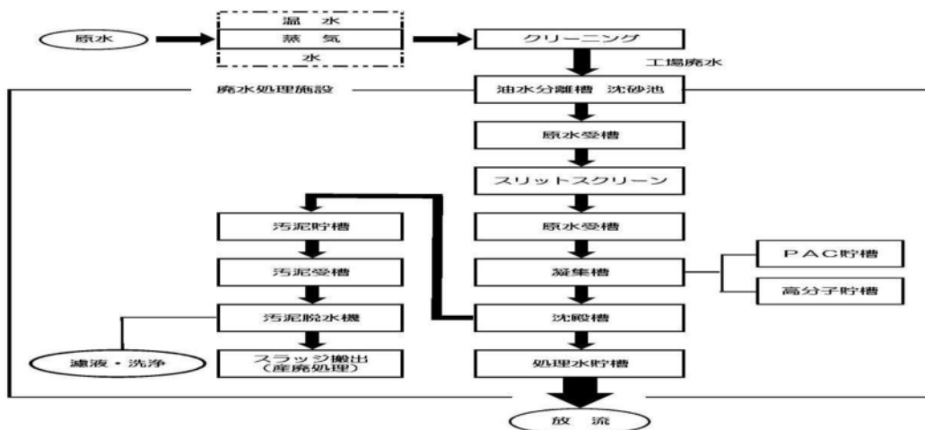
廃水処理方式
