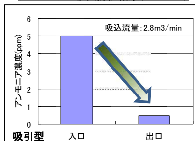
■ アンモニアの脱臭評価結果(ワンパス)
