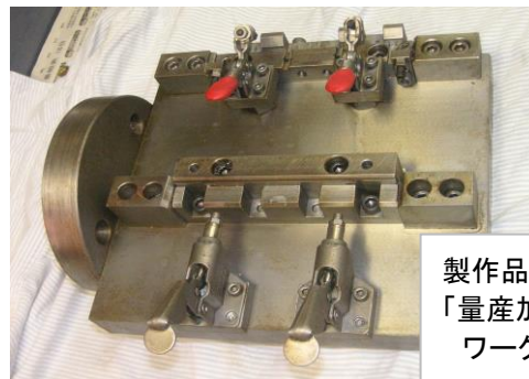
製作品例 「自動機用 ターンテーブル」
