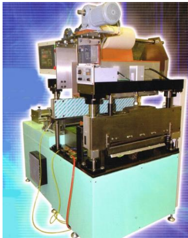
t0.05~0.5mm、幅600mm、 合紙挿入対応シャーリング装置
