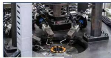
3 巻線
