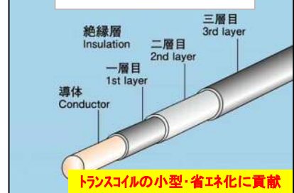
三層絶縁電線
