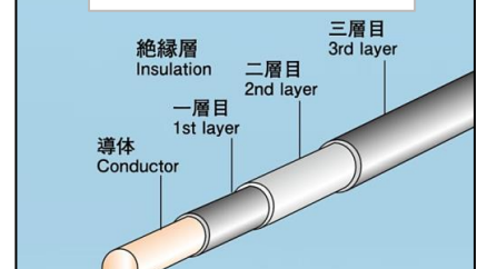
三層絶縁電線
