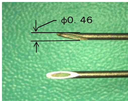
(製品仕様) φ0.46 × ℓ 28.448 材質SUS材
